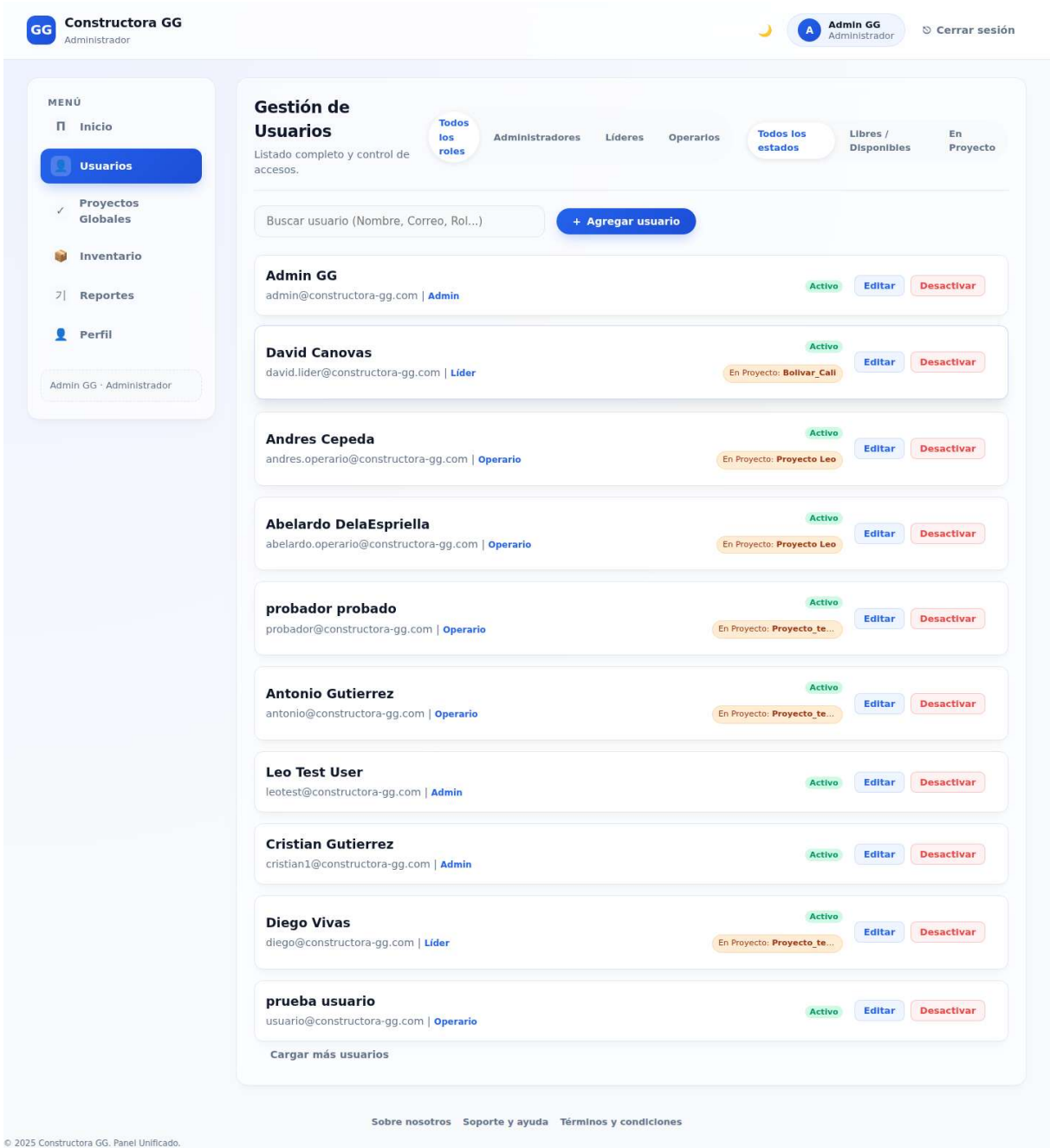
Listado de usuarios, con filtros por rol y por estado.
